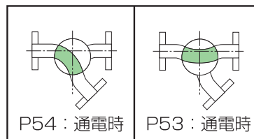
Y型3方弁 通電時流れ方向
