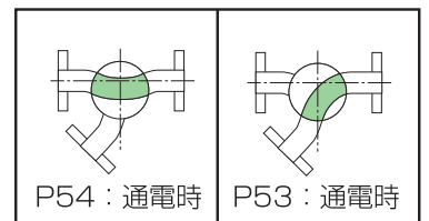
Y型3方弁 通電時流れ方向
